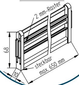
Längsteiler mit Rastenleiste & Teilerschuh
